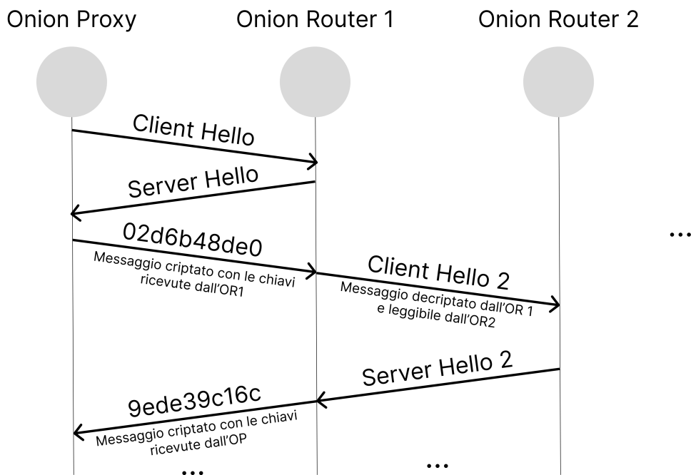
Figura 2.2: Creazione del circuito onion
