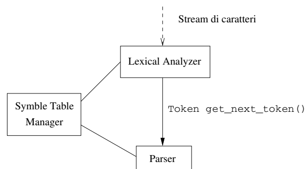
Figura 2.1: Interazioni dell'analizzatore lessicale.
