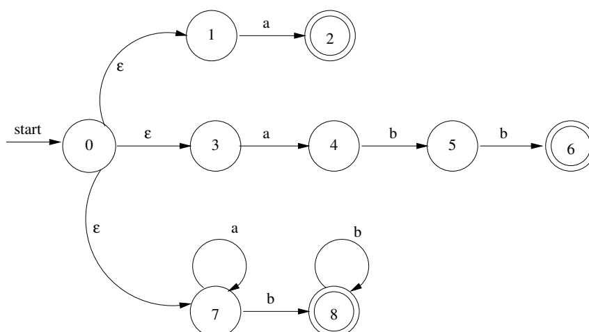
Figura 2.14: Un NFA che per il riconoscimento di tre pattern.
