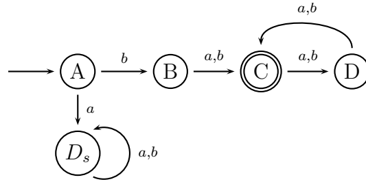
Figura 3.4: un DFA equivalente a r = b((a|b)(a|b))^*(a|b)
