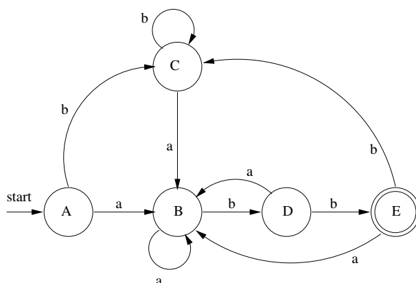
Figura 2.9: Un automa deterministico.
