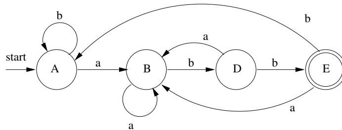
Figura 2.11: L'automa di Figura 2.9 minimizzato.
