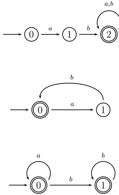
Figura 3.1: DFA equivalenti alle espressioni ab(a|b)^* , (ab)^* e a^*b^*
