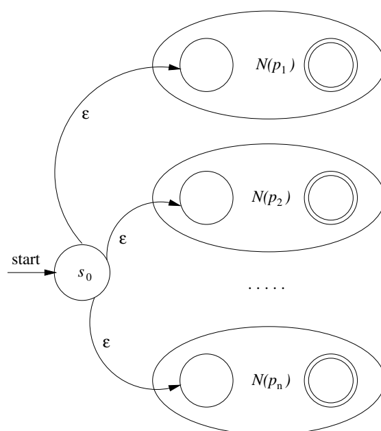
Figura 2.13: NFA usato per il pattern matching.
