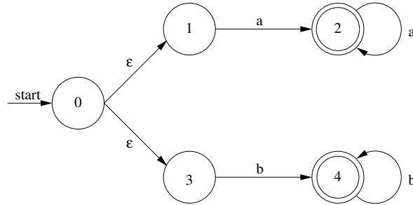
Figura 2.5: Un NFA contenente anche \epsilon -transizioni.
