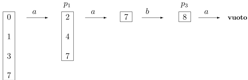
Figura 2.15: Sequenza di insiemi di stati attraversati leggendo l'input aaba .
