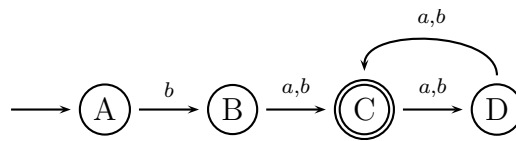
Figura 3.3: un DFA equivalente a r = b((a|b)(a|b))^*(a|b)
