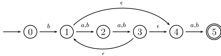
Figura 3.2: un possibile NFA equivalente a r = b((a|b)(a|b))^*(a|b)
