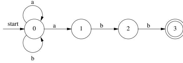
Figura 2.4: Un NFA.
