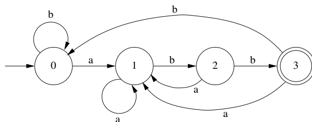
Figura 2.6: Un automa deterministico.
