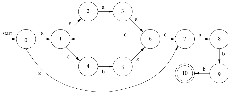
Figura 2.8: Un automa non deterministico per (a|b)^*abb .
