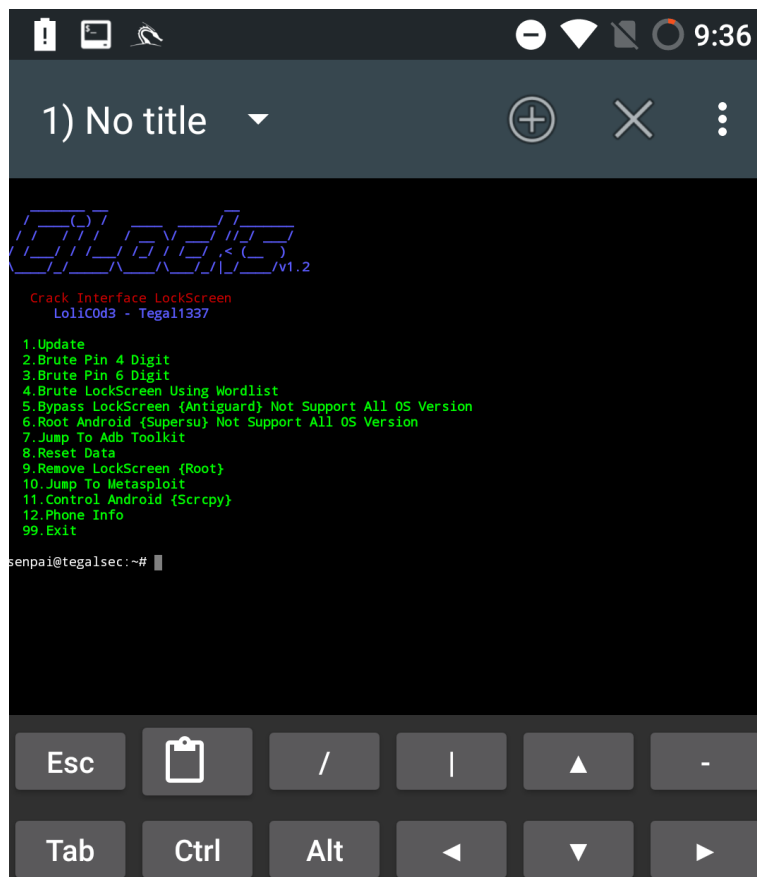
Figura 4.6: CiLocks esempio
