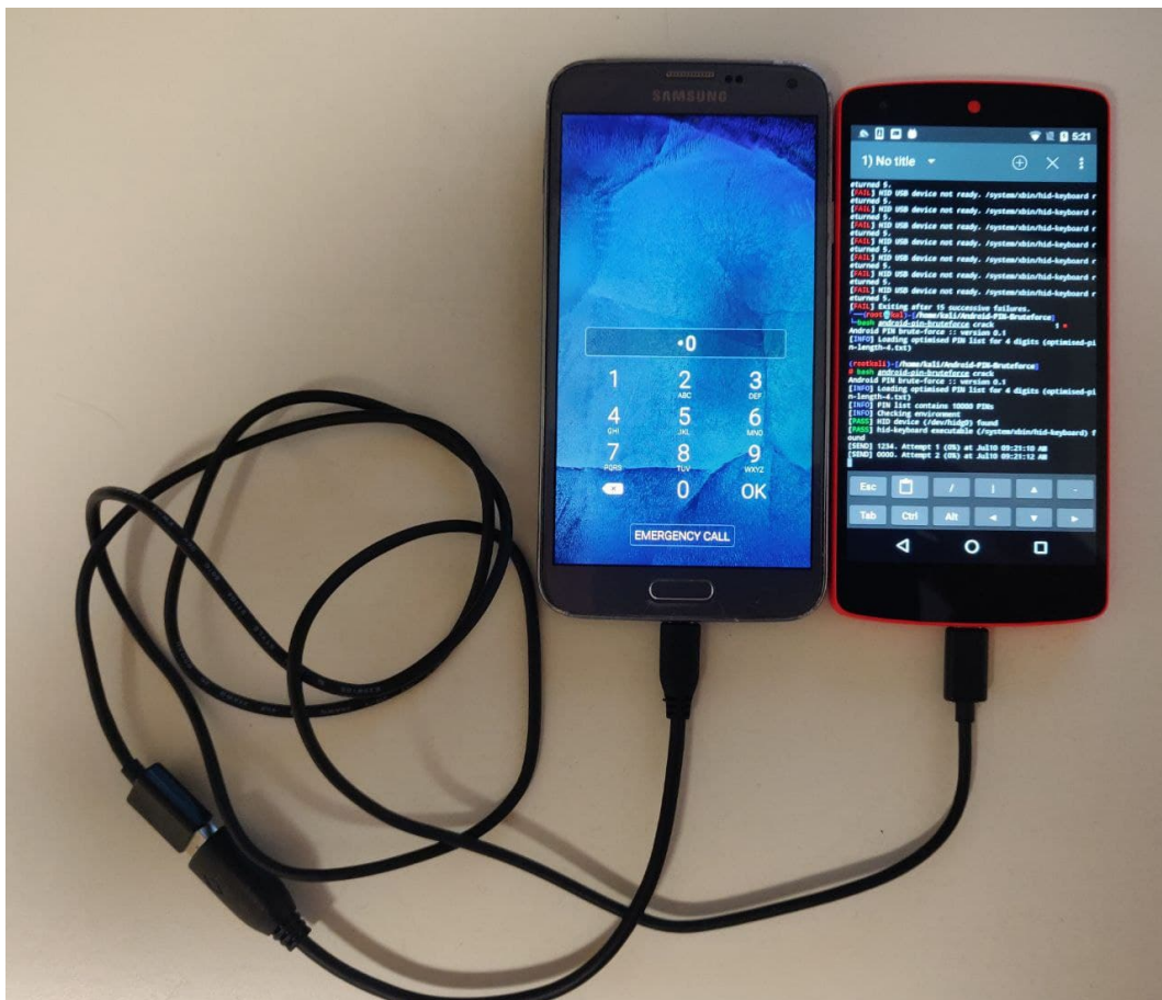
Figura 4.3: Android-PIN-Bruteforce esempio
